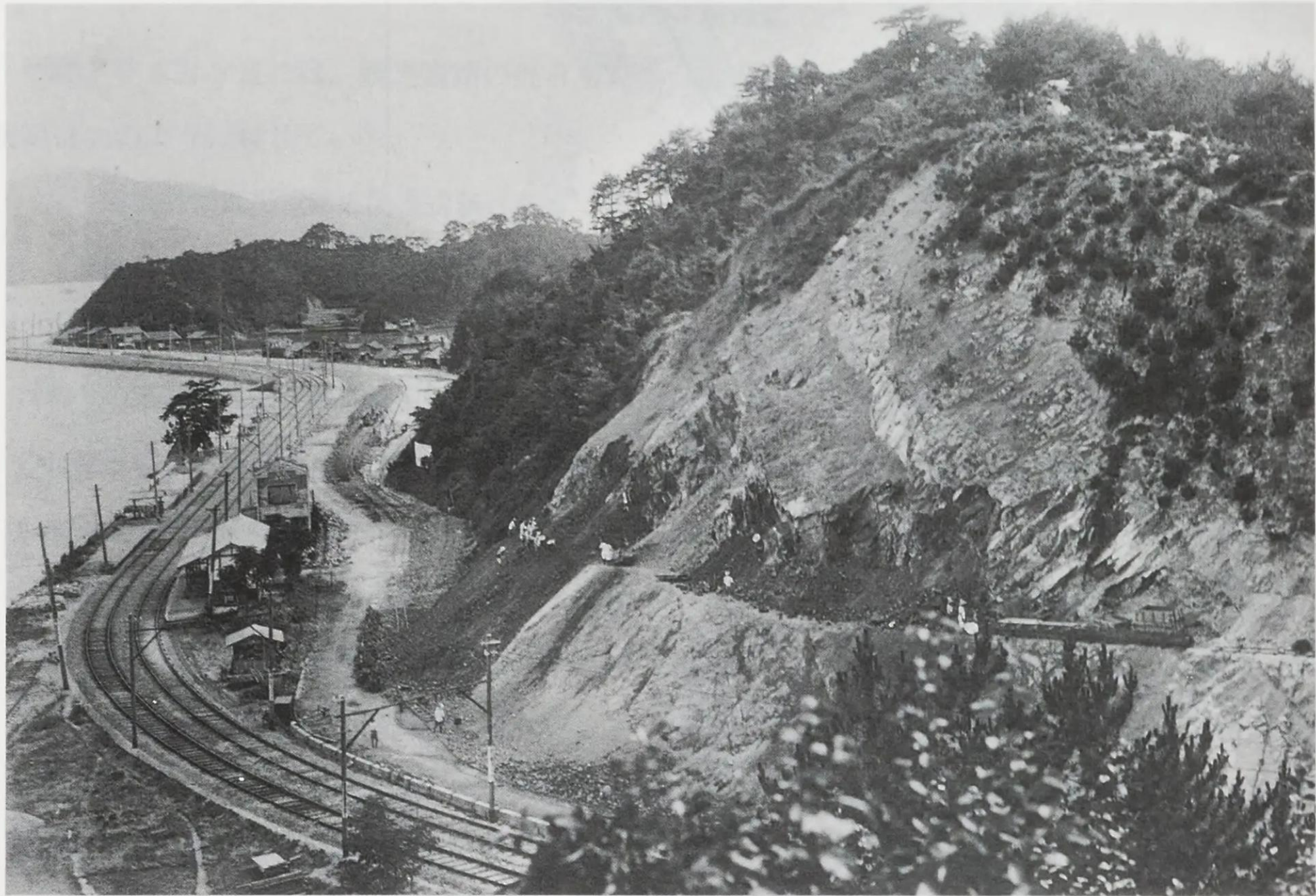
廿日市町地御前取付工事(昭和6年7月)
